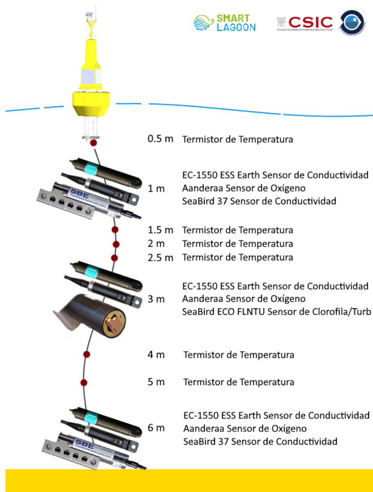
Figura 18: Esquema de los sensores instalados en la boya piloto SMLG con los nuevos sensores de temperatura, conductividad y presión a 1 y 6 metros de profundidad (Seabird-37).
