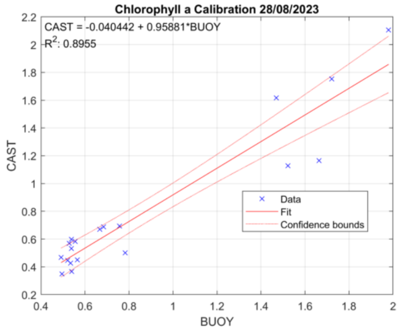
Figura 26: Calibración de la fluorescencia de la boya SMARTLAGOON con la Clorofila a obtenido de la fluorescencia del CTD.
