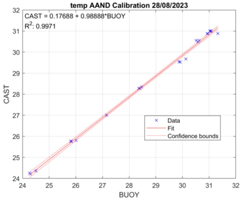
Figura 22: Calibración de los datos de temperatura de los sensores de oxígeno Aanderaa de la boya SMLG - 14/07/2023 a hoy.
