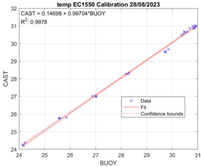
Figura 24: Calibración de la temperatura del sensor de conductividad (EC-1550) de la boya SMLG - 14/07/2023 a hoy.
