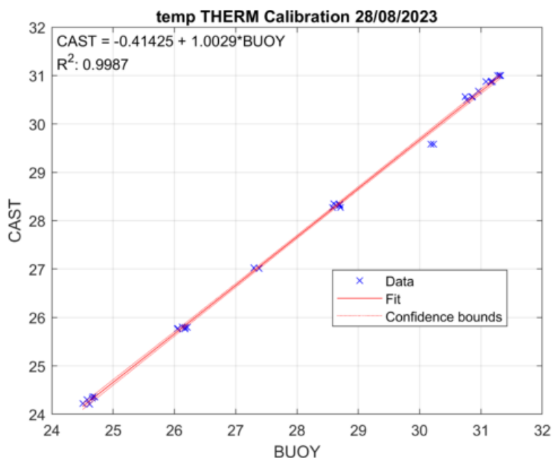
Figura 20: Calibración de los datos de temperatura de los Termistores de la boya SMLG - 14/07/2023 a hoy.
