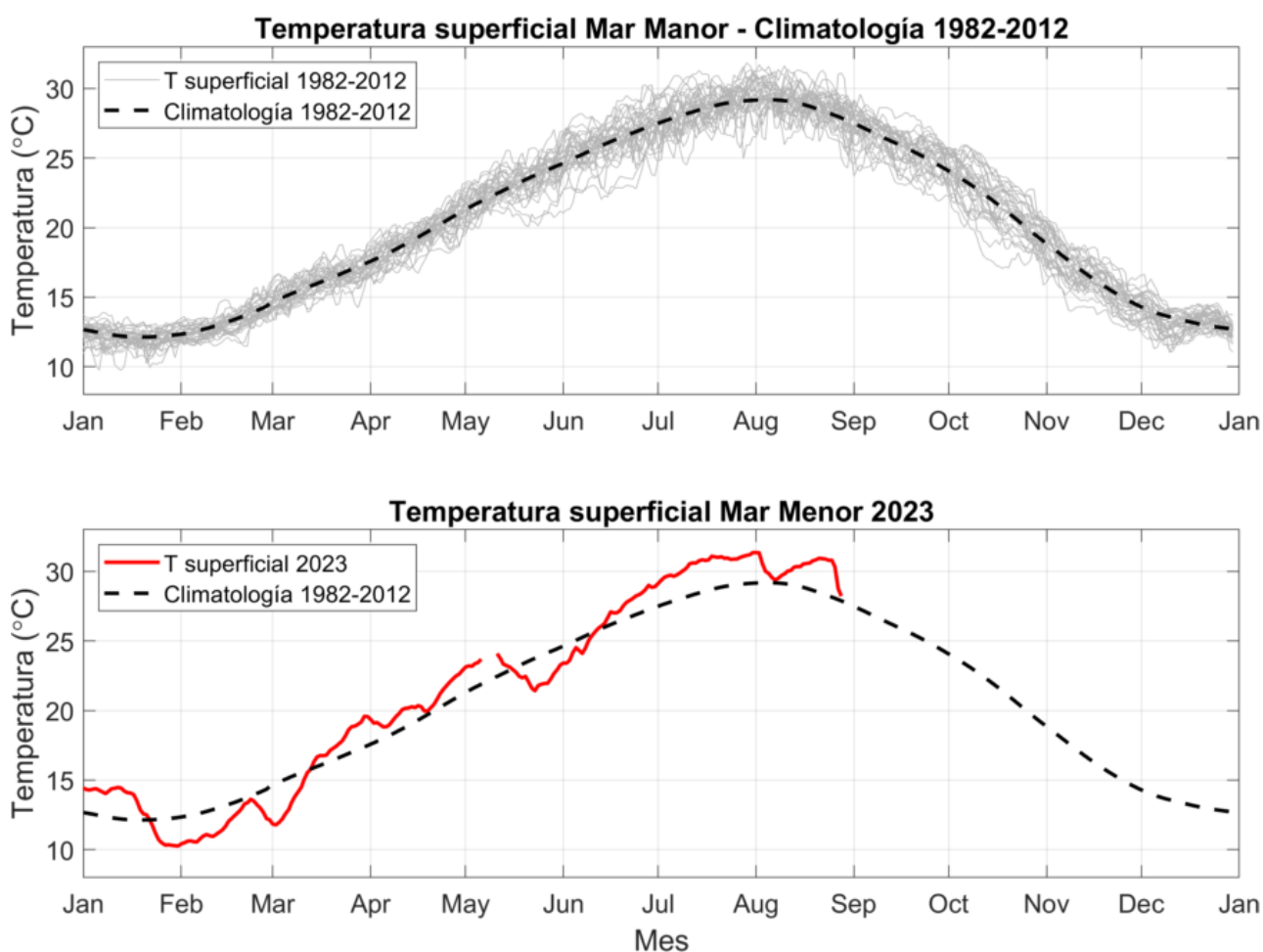
Figura 5: Serie temporal de temperatura obtenida a cada profundidad por los sensores de la boya SMLG, calibrados con los datos de CTD obtenidos por el IEO-CSIC. 5a: la serie climatológica utilizada como referencia para el análisis de olas de calor (1982-2012). 5b: Serie de temperatura comparada con la serie climatológica de referencia
